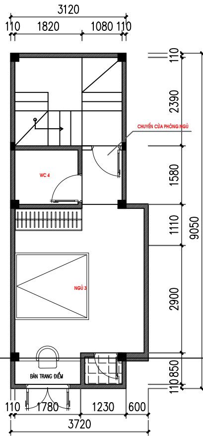
MẶT BẰNG NỘI THẤT T.3
