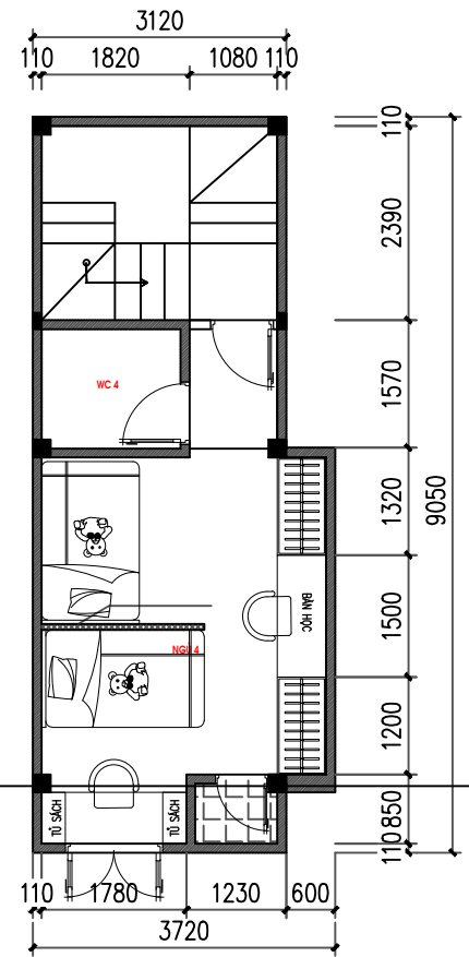
MẶT BẰNG NỘI THẤT T.4
