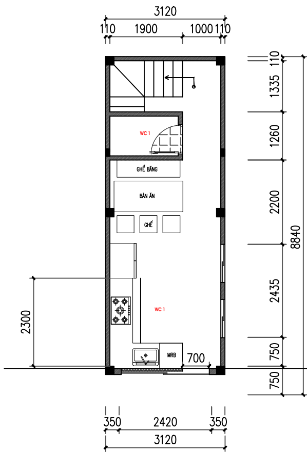
MẶT BẰNG NỘI THẤT T.2
