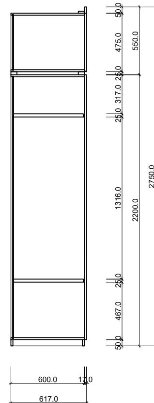
MẶT CẮT 3-3
