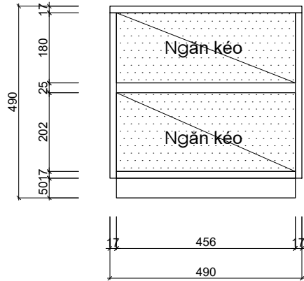
MẶT ĐỨNG
