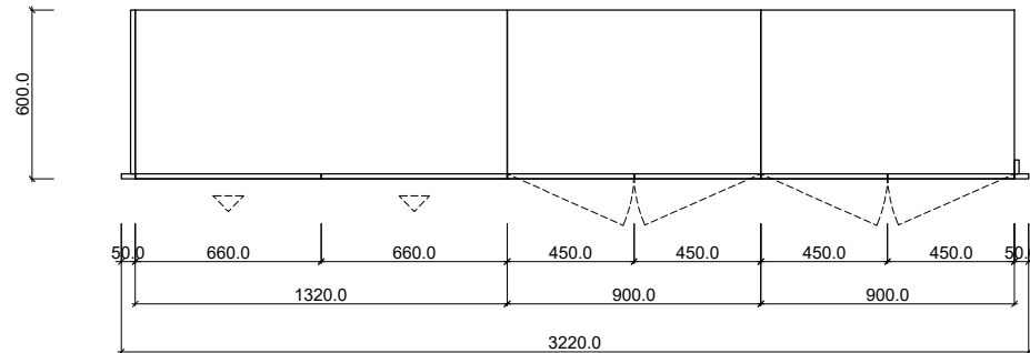
MẶT BẰNG
