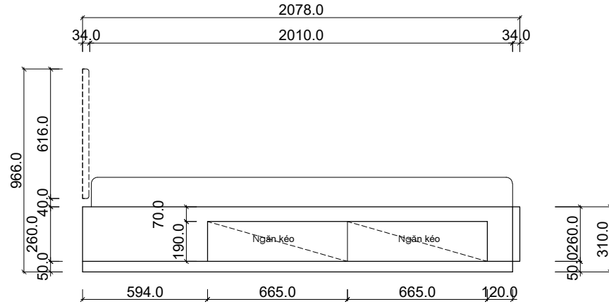
MẶT BÊN
