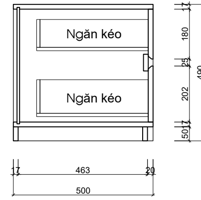
MẶT CẮT BÊN
