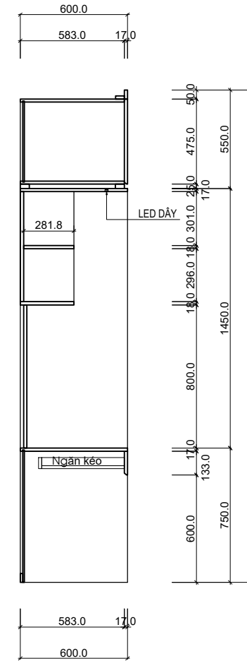
MẶT CẮT 2-2
