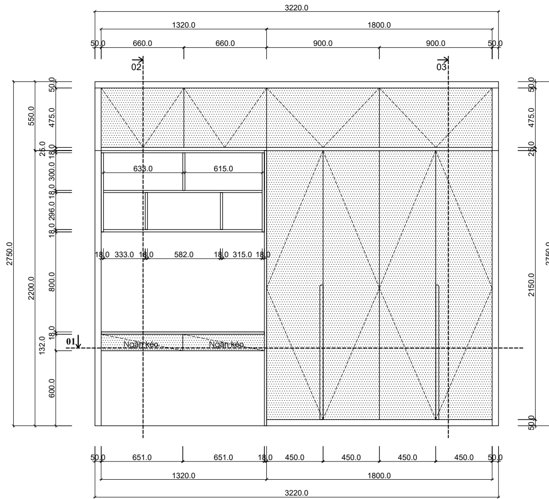
MẶT ĐỨNG
