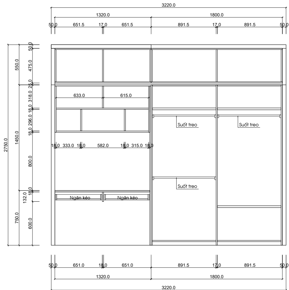
MẶT ĐỨNG BỎ CÁNH
