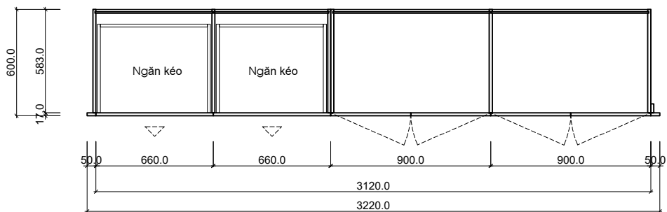
MẶT CẮT 1-1
