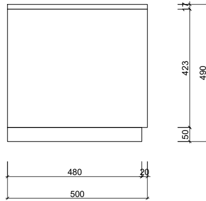
MẶT BÊN
